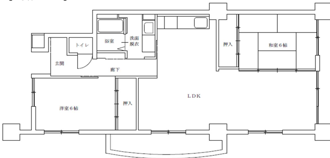
【3号棟：2LDK】
